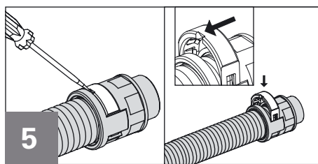
To re-open use a screwdriver. The screwdriver slot at the oval clip (C) must point towards the conduit. Wieder öffnen mittels Schraubenzieher. Die Schraubenzieher-Öffnungsnut an der Sperre (C) muss rohrrseitig positioniert sein.
