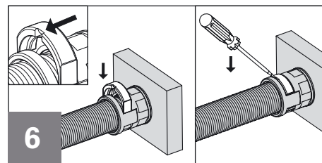
Insert Oval clip (D) in the locking element window and click into place. The screwdriver slot must point towards the conduit. To re-open use a screwdriver. Oval-Sperre (D) in das Sperrenfenster einsetzen und einrasten. Die Schraubenzieher-Öffnungsnut muss rohrrseitig positioniert sein. Wieder öffnen mittels Schraubenzieher.
