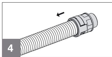
Pull back the conduit (A) slightly to ensure the locking mechanism is fully engaged. Wellrohr (A) leicht zurückziehen, damit die Verriegelungselemente optimal einrasten.
