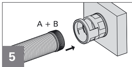
Push conduit with seal cap (A+B) into the fitting until seal cap is no more visible in the locking element window. Rohr mit Dichtkappe (A+B) so weit in den Fitting einstossen, dass die Dichtkappe nicht mehr im Sperrenfenster sichtbar ist.
