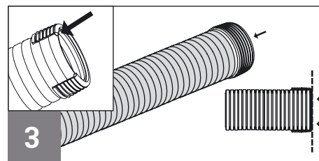
Push seal cap (B) completely onto conduit in order to achieve IP68. Für Schutzart IP68 Rohrdichtung (B) ganz auf das Rohr aufstossen.
