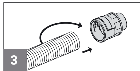
Push in the conduit (A) with a slight twist until the stop. Einstossmontage des Wellrohres (A) mit leichter Drehbewegung. Rohr bis zum Anschlag einstossen.
